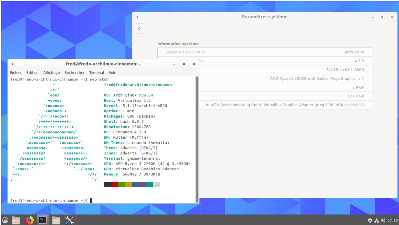
Illustration 18 : Cinnamon 4.2.0
